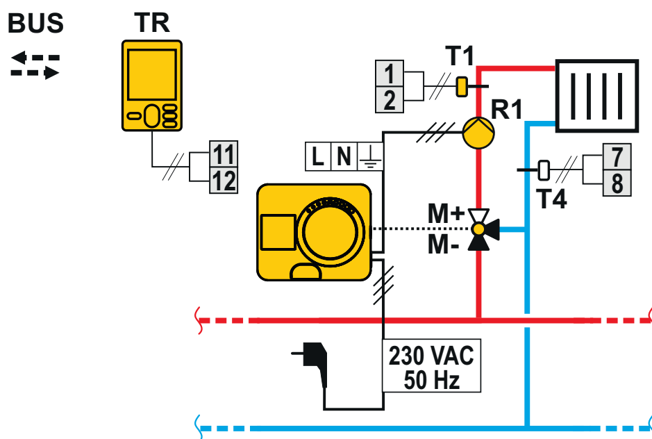
SCHÉMA 360B - circuit de chauffage supplémentaire
