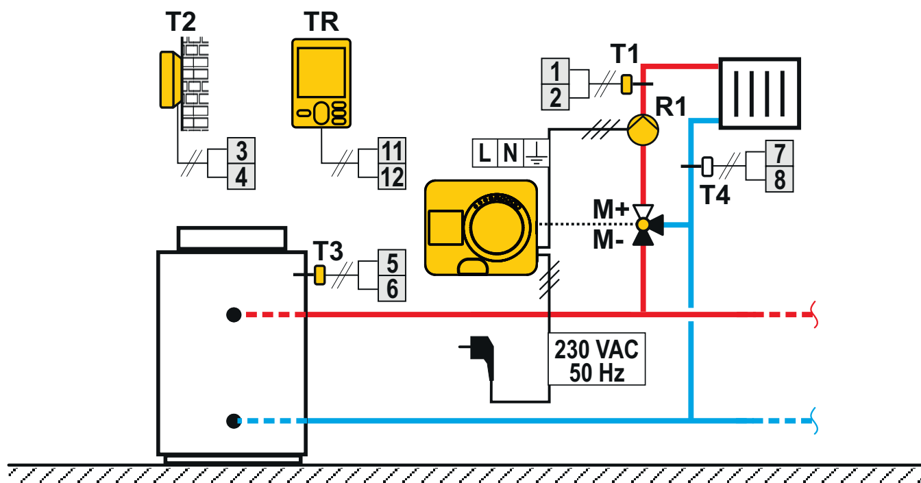
SCHÉMA 360 - circuit de chauffage
